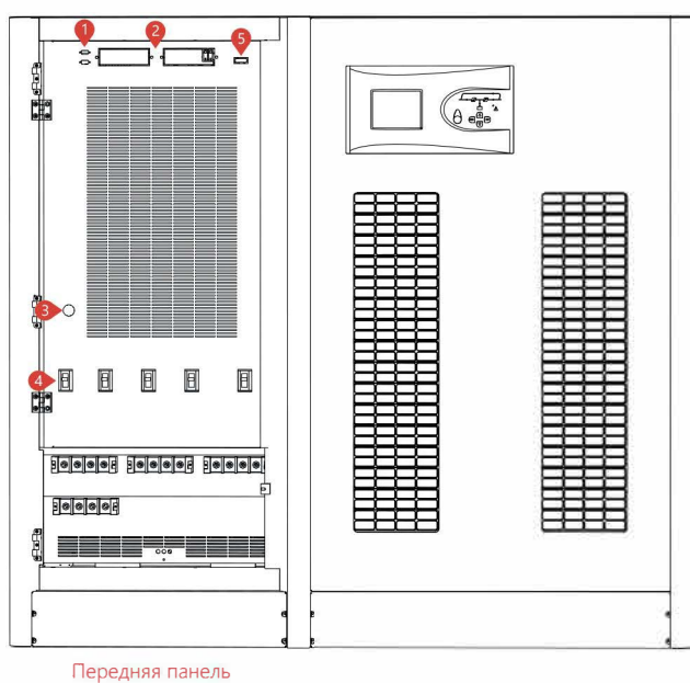
Передняя панель
