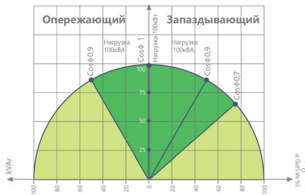
LevelUps Диаграмма выходного фактора мощности
