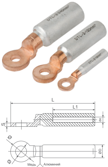
Медно-алюминиевые соединительные клеммы DTL-2
