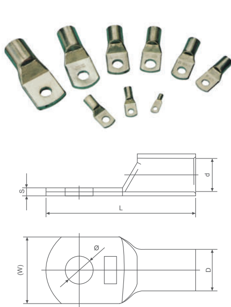
Медные клеммы SC(JGK)
