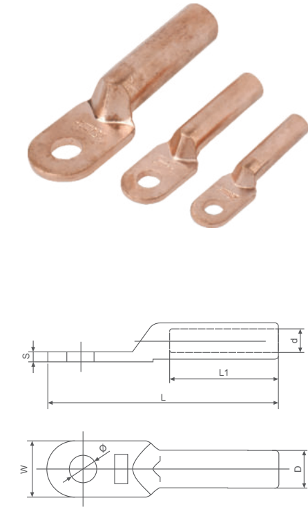
Медные соединительные клеммы DT
