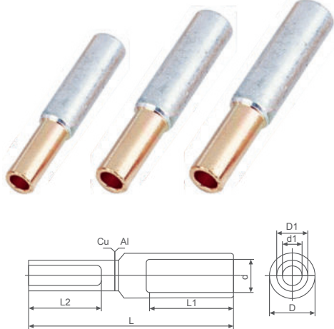
Медно-алюминиевая соединительная трубка GTL (с
