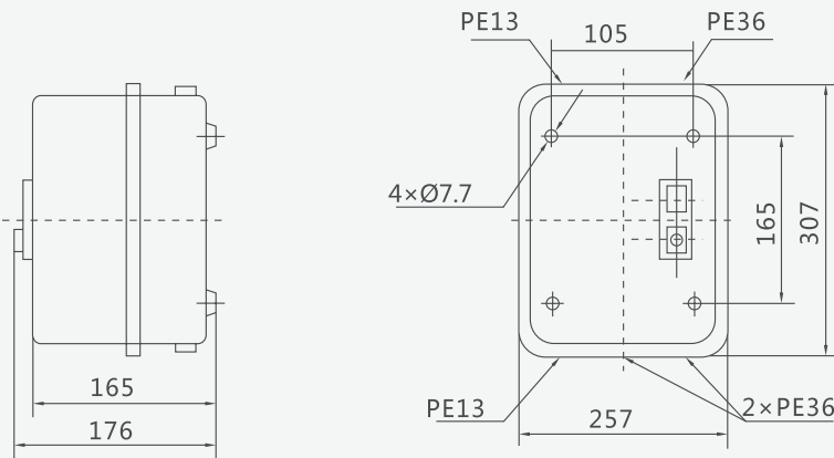
LE1-D40, D50, D65, D80, D95
