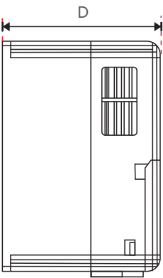
Рисунок А-1. Габаритные размеры для моделей мощностью до 7,5 кВт (380 В)
