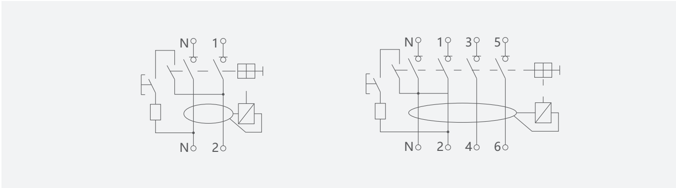
Схема подключения
