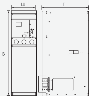
442×845×1550(Ш*Г*В) ячейка для подъема (перемещения)
