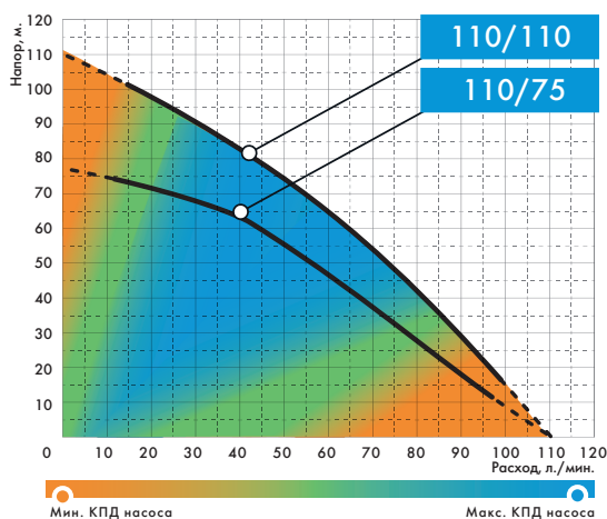
График расходно-напорных характеристик*:
