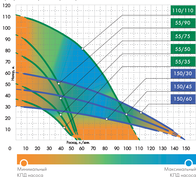
График напорных характеристик*:
