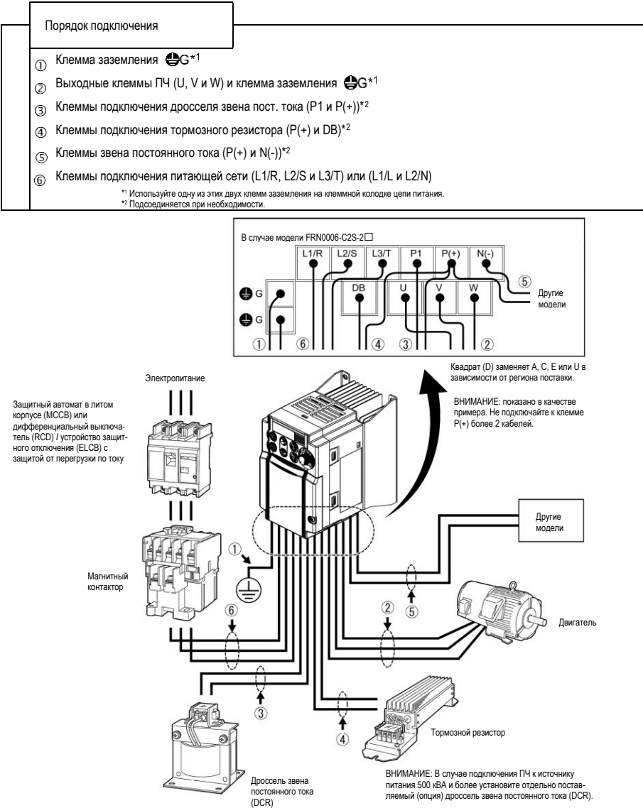
Рисунок 2.3 Порядок подключения периферийного оборудования
