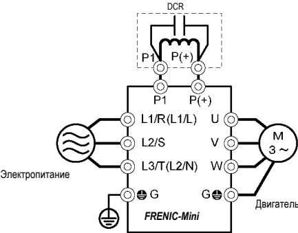
Рисунок 10.1 Схема соединений дросселя звена постоянного тока (DCR)
