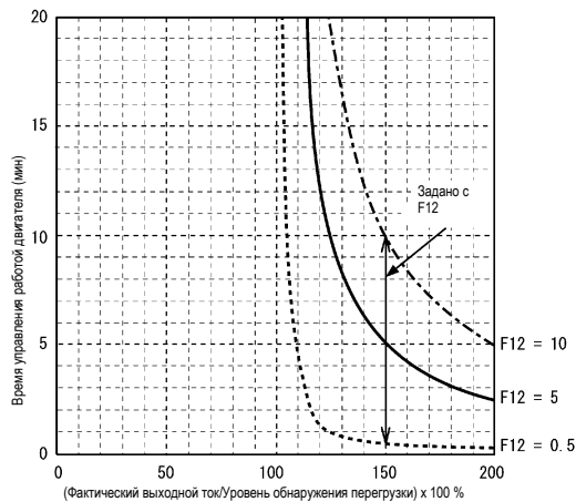
Пример характеристики обнаружения тепловой перегрузки
