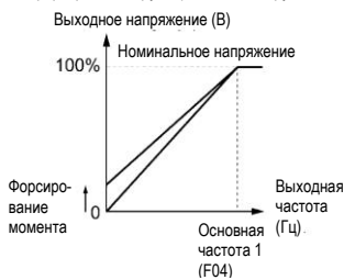
Линейная модель V/f (F37 = 1)
