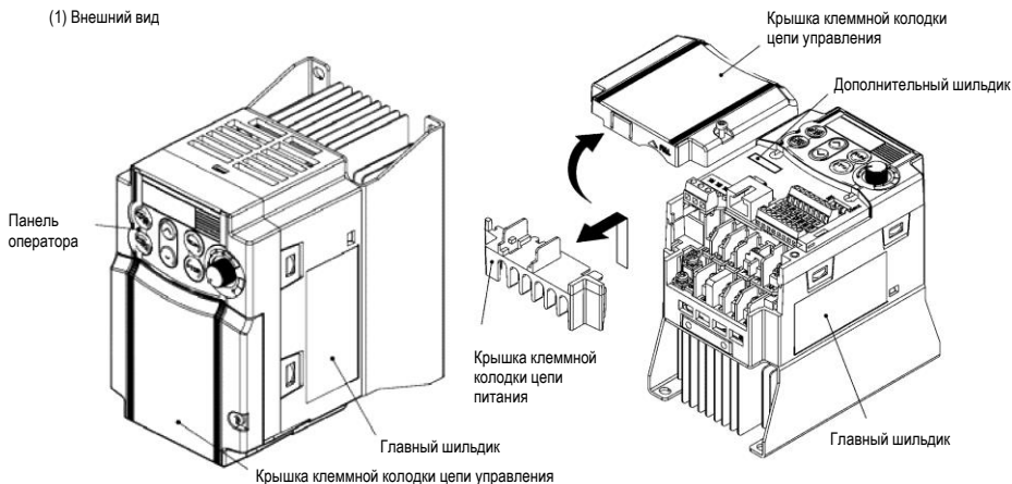
Рисунок 1.2. Внешний вид FRENIC-Mini
