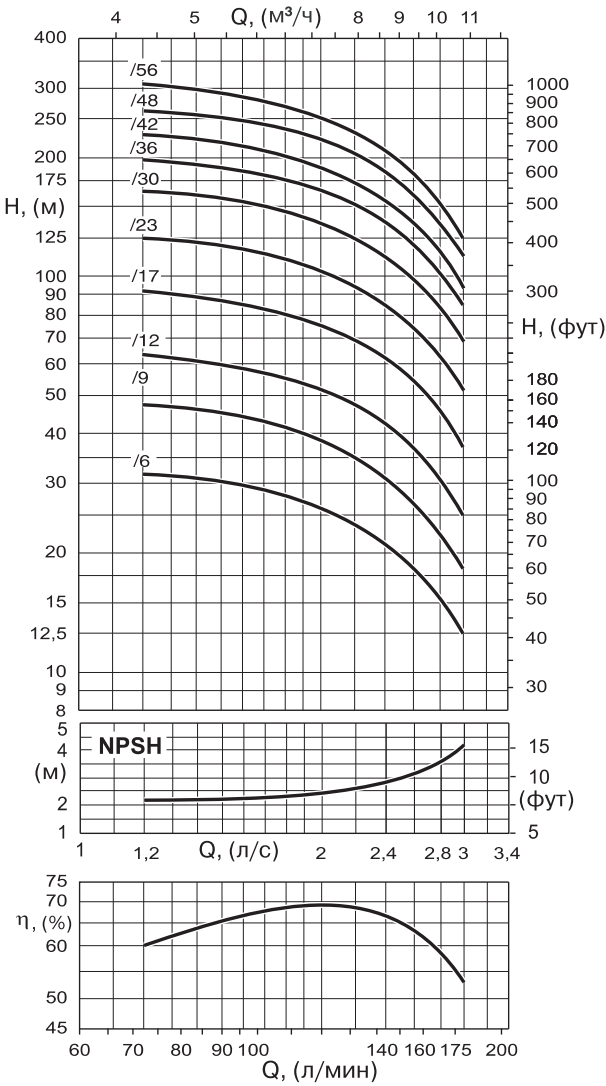
Эксплуатационные характеристики для насосов с 2-полюсными электродвигателями, частота 50 Гц
