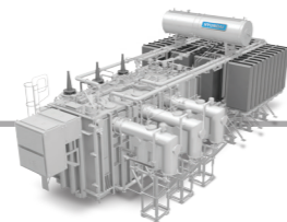
Силовой трансформатор • до 800 кВ, 1500 МВА
