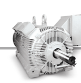
Электродвигатель серии Н + С • 150-1300 л.с. • 2000-7200 В, 50/60 Гц • 2-8 полюсов
