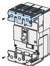
Схема сборки
