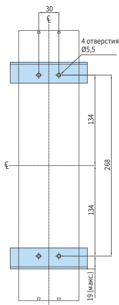
Монтажный чертёж
