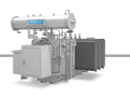
Силовой трансформатор • 800 кВ, 1500 МВА
