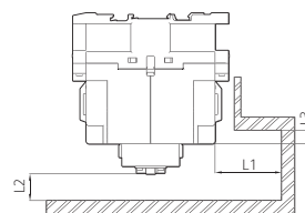
Изоляционное расстояние
