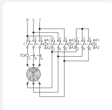
Схема главной цепи
