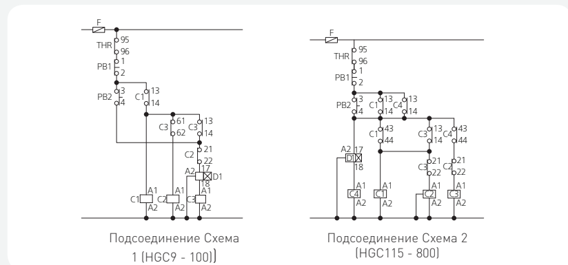
Цепь управления
