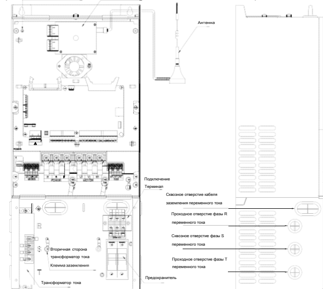
Вид интегрированной машины спереди
