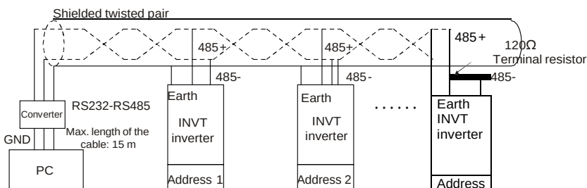
Рис 9.4 Практическая схема
